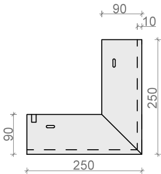
NAROŻNIK ZEWN. 90° NK 95ALz, NK 95Sz
