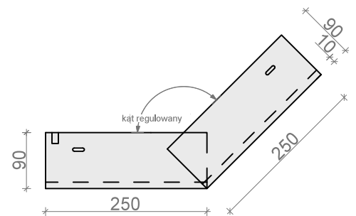
NAROŻNIK ZEWN. regulowany NK 95ALzR, NK 95SzR
