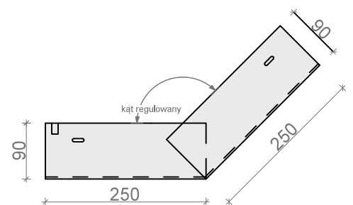
NAROŻNIK ZEWN. regulowany NK 55ALzR, NK 55SzR
