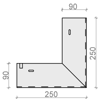
NAROŻNIK ZEWN. 90° NK 55ALz, NK 55Sz
