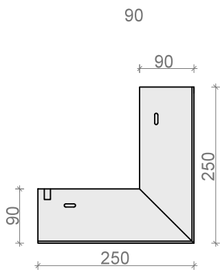
NAROŻNIK ZEWN. 90° NKP 10ALz, NKP 10Sz
