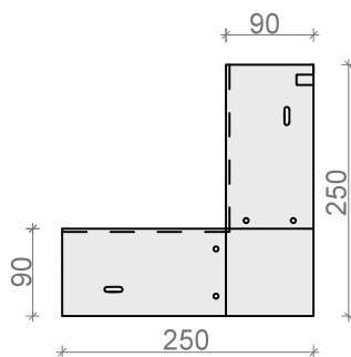
NAROŻNIK WEWN. 90° NK 30ALw, NK 30Sw
