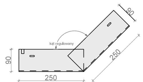
NAROŻNIK ZEWN. regulowany NK 30ALzR, NK 30SzR
